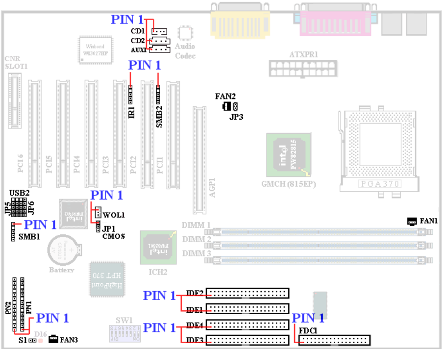
圖 2-7. ST6/ST6-RAID 所有的連接埠及接頭
