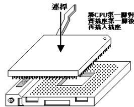
圖2-4. 將處理器安裝到Socket 370插座
