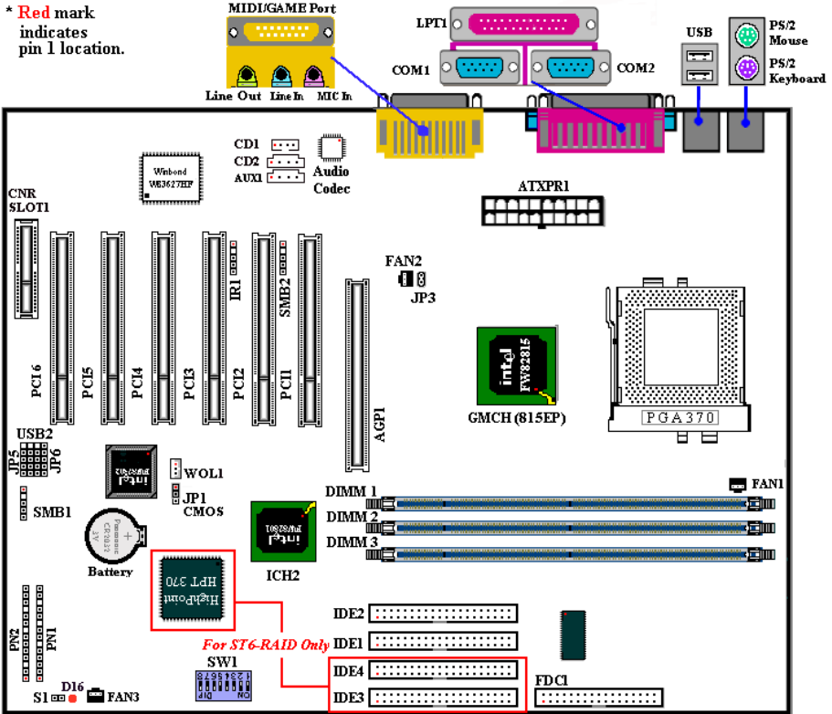
圖 1-1. ST6/ST6-RAID 主機板重要元件位置圖
