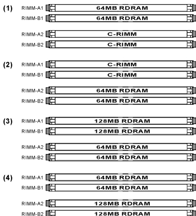
圖 2-5. 記憶體模組組態範例
