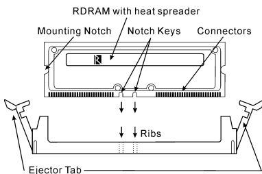
圖 2-6. 記憶體模組的安裝
