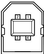
针脚配置
