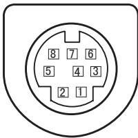
针脚配置
