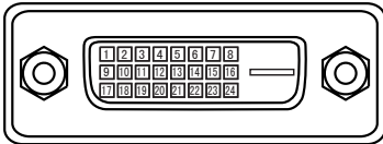
针脚配置
