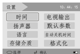
设置界面
