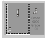
俄罗斯方块
