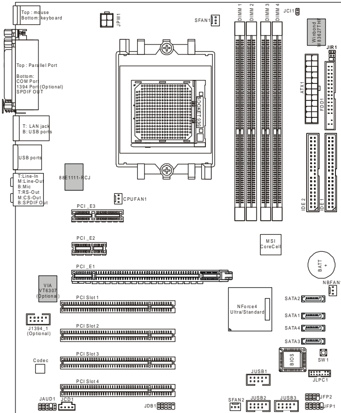
K8N Neo4 系列 (MS-7125) v1.X ATX 主機板
