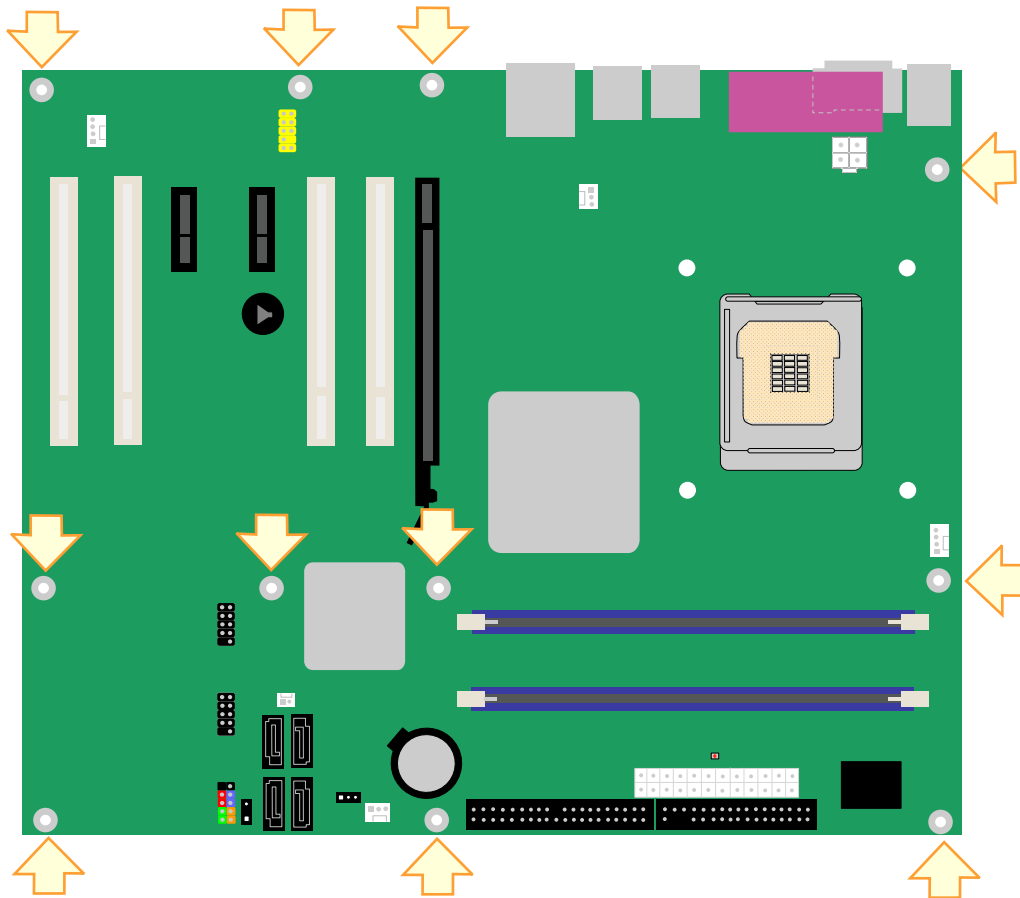
图 5. 台式机主板 D945PLRN 安装螺丝孔位置
