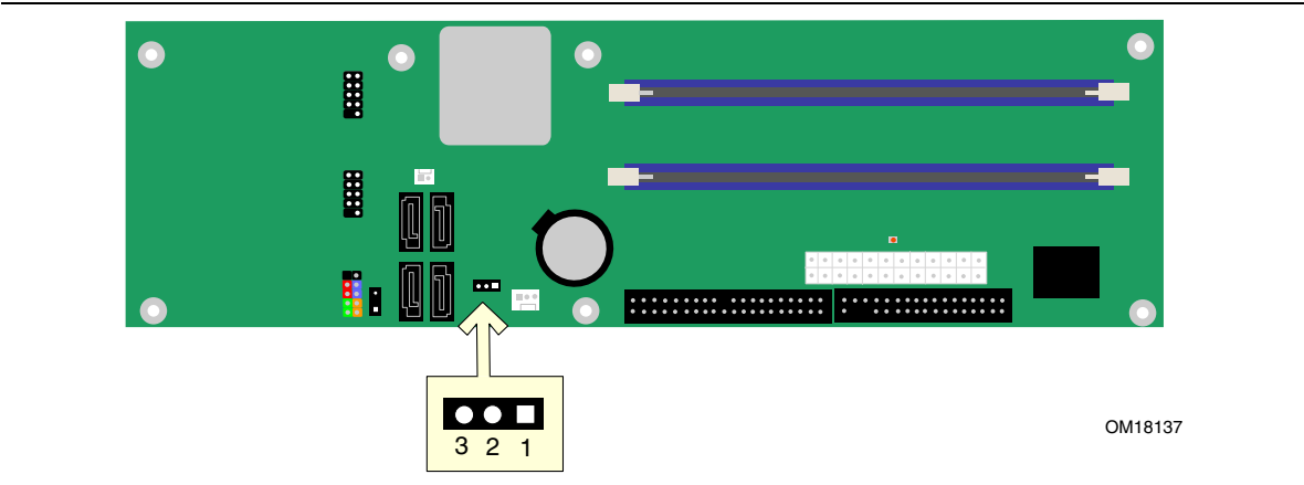
图 23. BIOS 配置跳线位置
