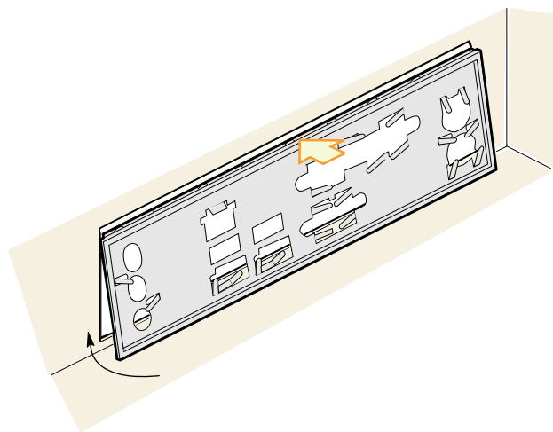
图 4. 安装 I/O 防护板
