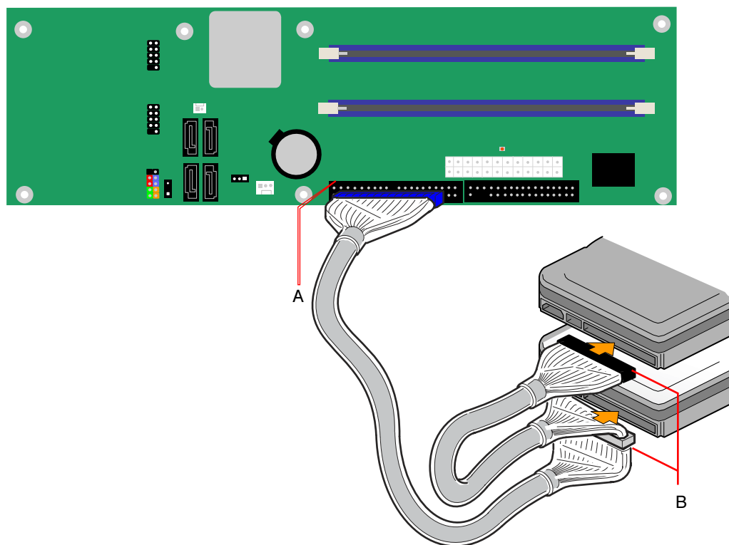
图 16. 连接 IDE 电缆
