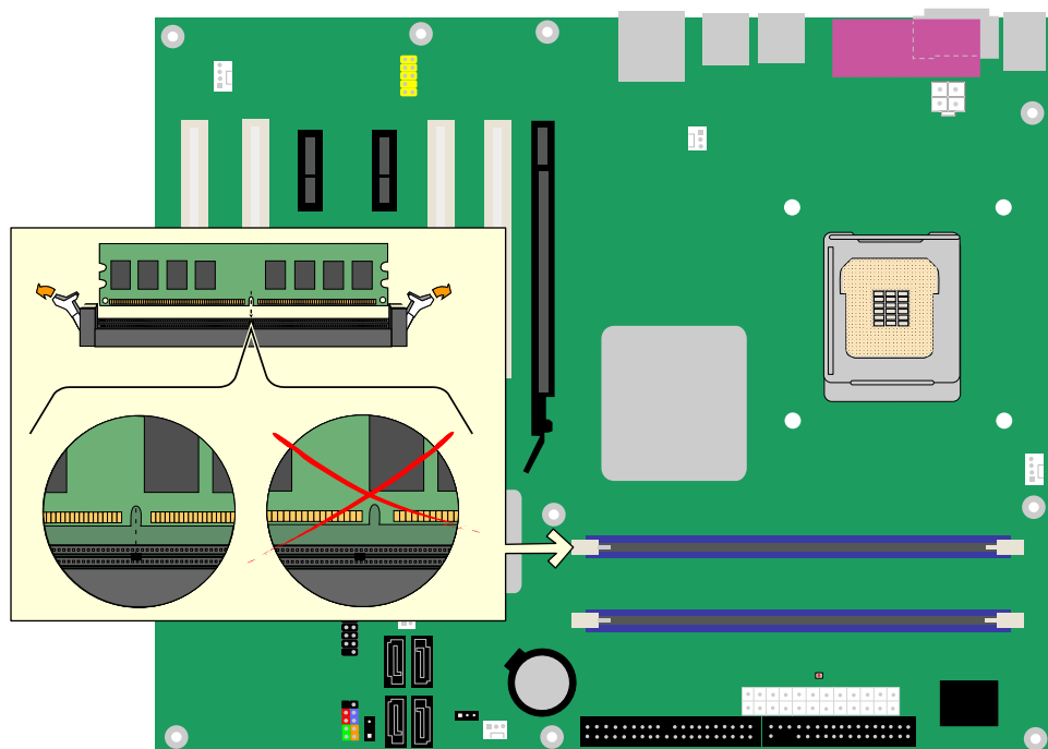
图 14. 安装 DIMM
