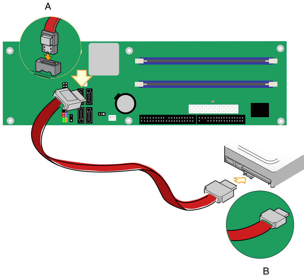
图 17. 连接串行 ATA 电缆
