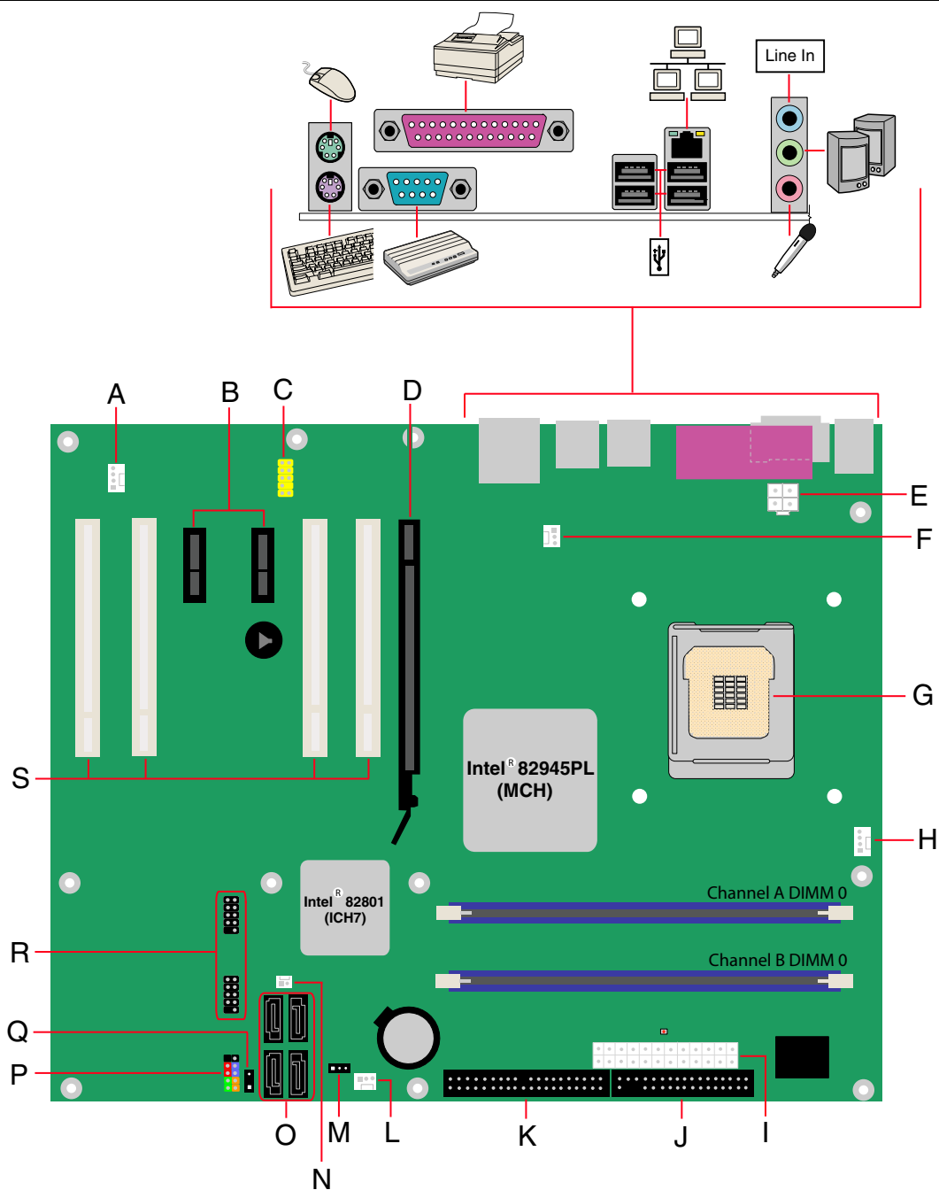
图 1. 台式机主板 D945PLRN 组件
