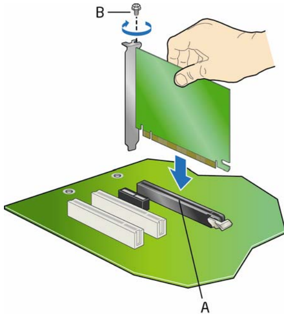
图 18. 安装 PCI Express x16 卡
