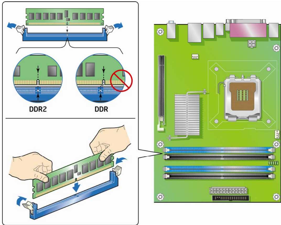
图 17. 安装 DIMM
