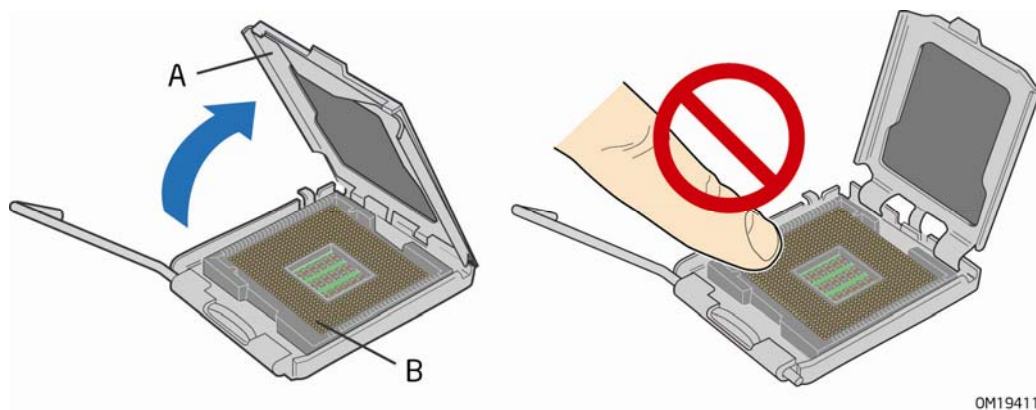
图 7. 抬起压板
