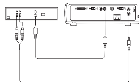
连接 S-video（超级视频）和音频线
