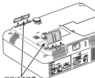
空气过滤装置 拔出并取下。
