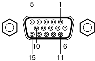
微型D-sub 15针连接器
