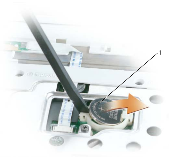
1 币形电池
