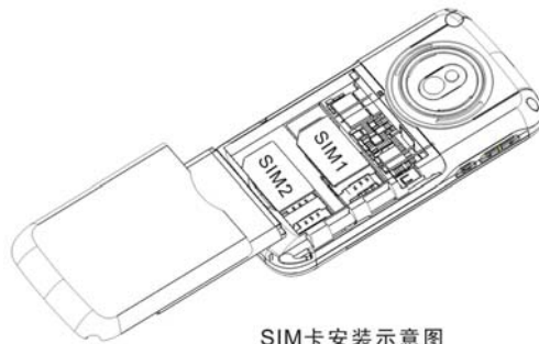
SIM卡安装示意图
