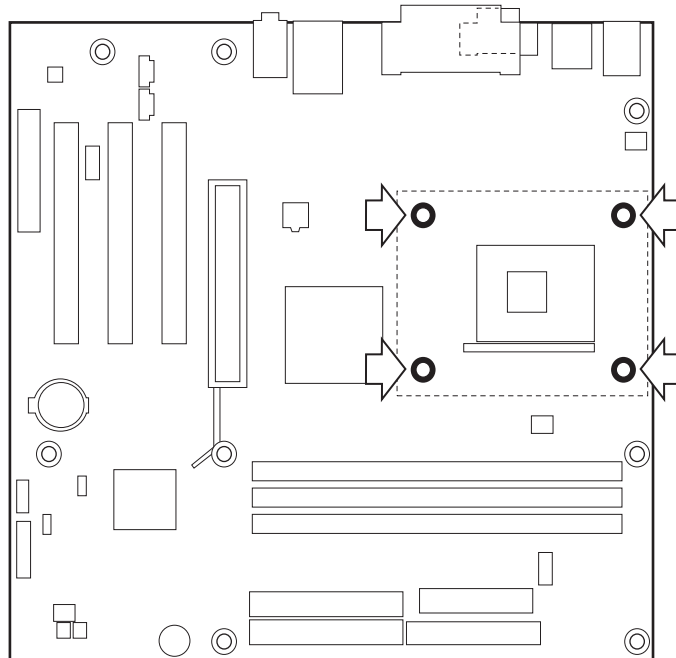
图 7. 处理器风扇散热器固定架安装孔位
