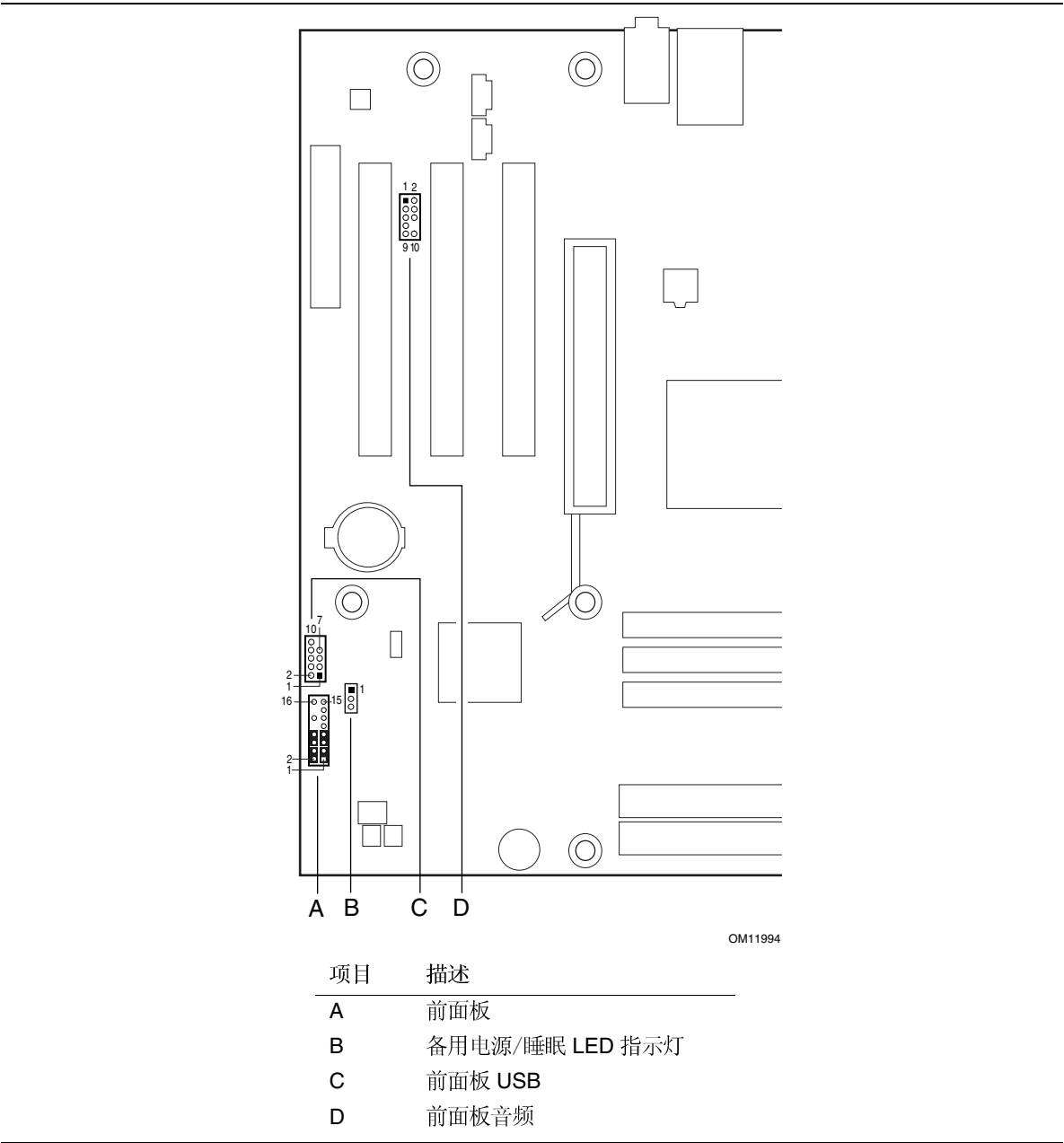
图 24. 前面板连接器
