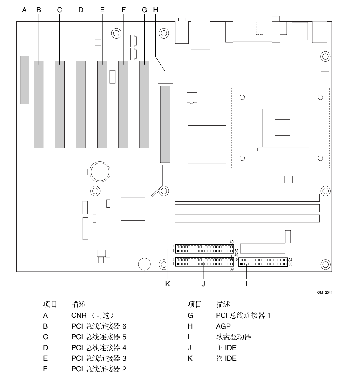
图 23. D845WN 母板的附加卡和外围设备接口连接器
