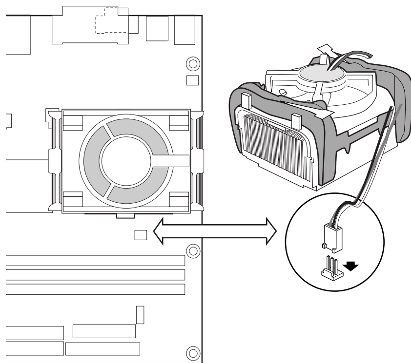
图 10. 将处理器风扇散热器电缆连接到处理器风扇连接器上
