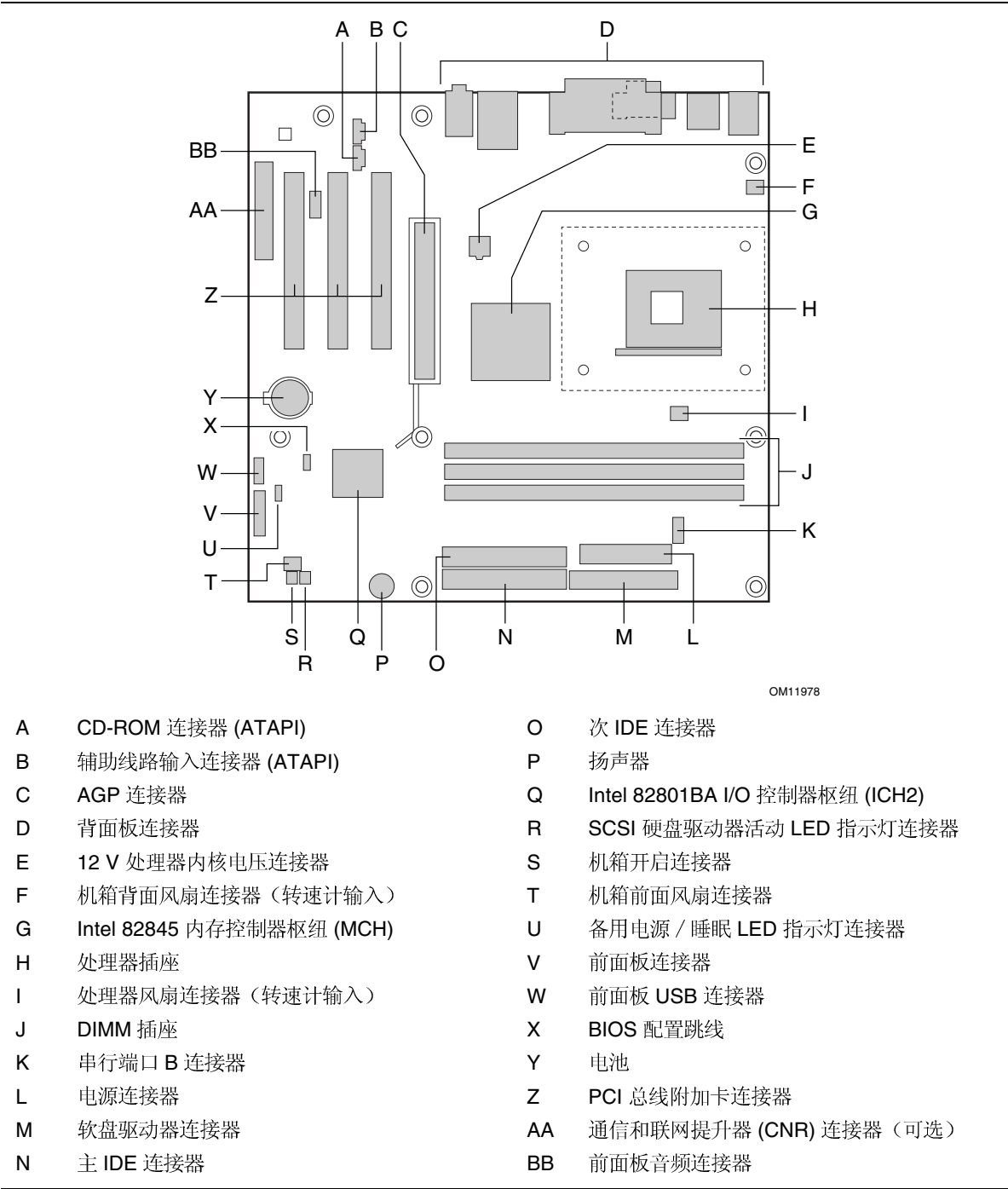
图 1. D845HV 桌面主板元件
