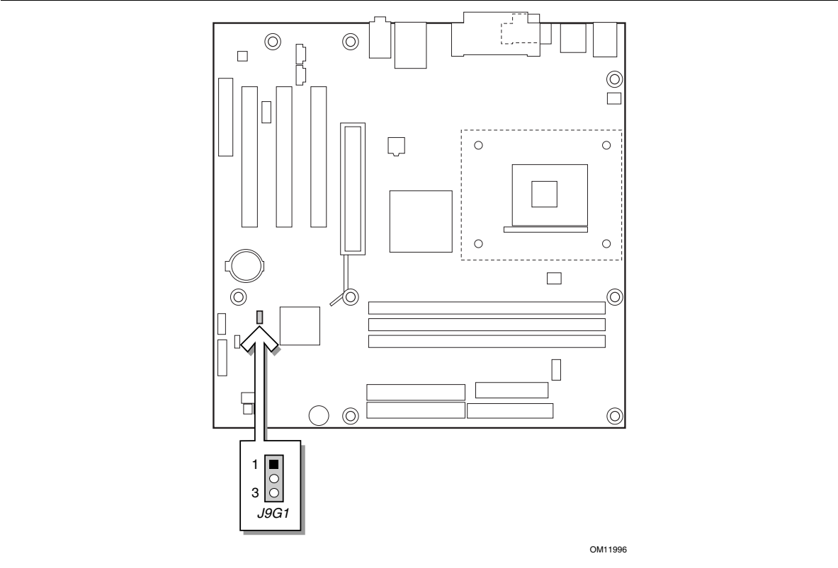
图 17. BIOS 配置跳线块的位置
