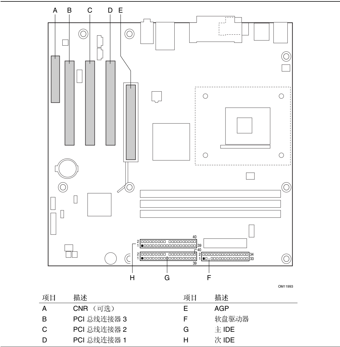
图 22. D845HV 母板的附加卡和外围设备接口连接器
