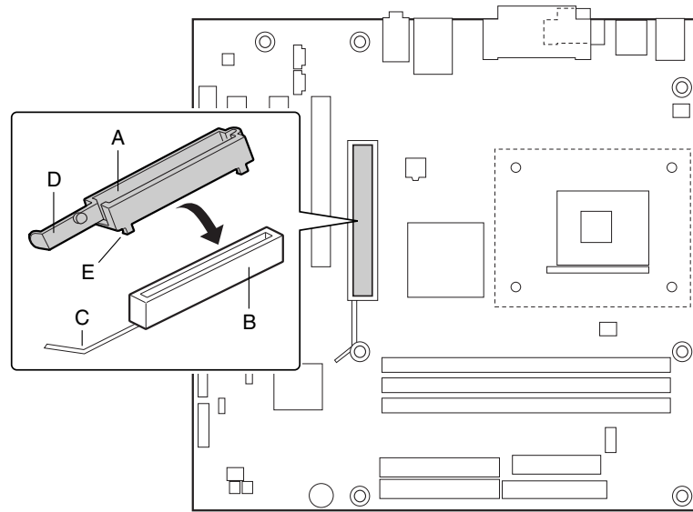
图 13. 安装 AGP 卡固定架
