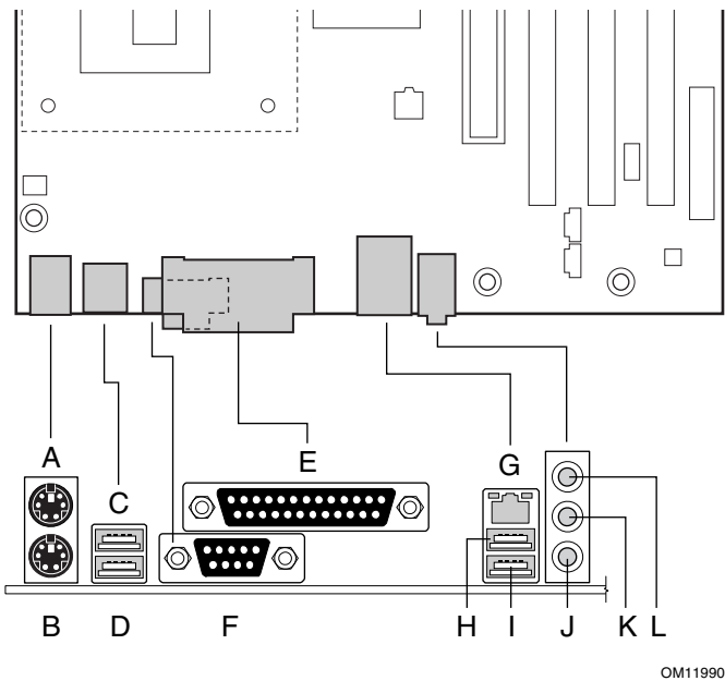
图 19 显示桌面主板上的背面板连接器。
