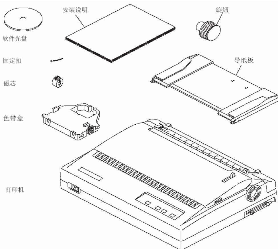
图 1-1 开箱示意图
