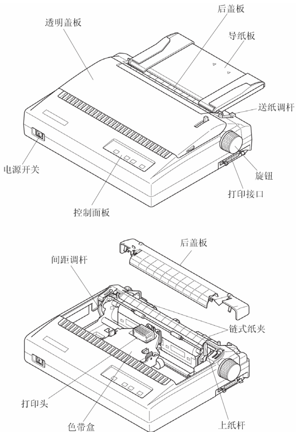
图 1-2 打印机外型示意图
