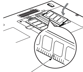
模塊內槽口
